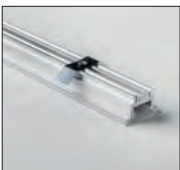
Molla a pressione Foro incasso larghezza 20 mm - Altezza 14 mm Posizionare inizio-fine +1 ogni 50 cm. Spring for recessed ceiling. Recessed hole width 20 mm - Height 14 mm. Place: beginning, end and 1 every 50 cm
